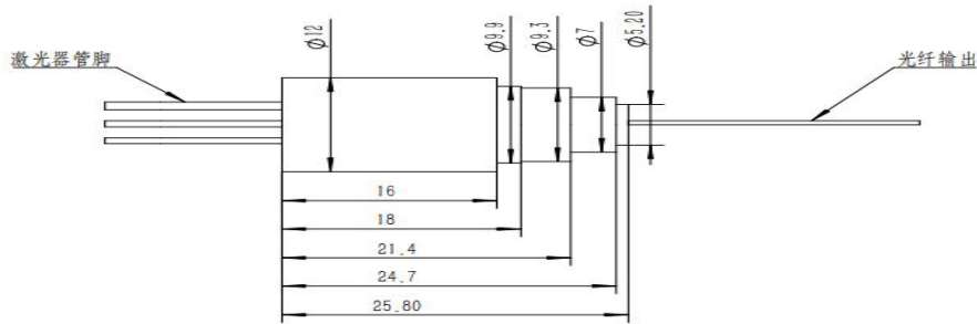
同轴封装图
